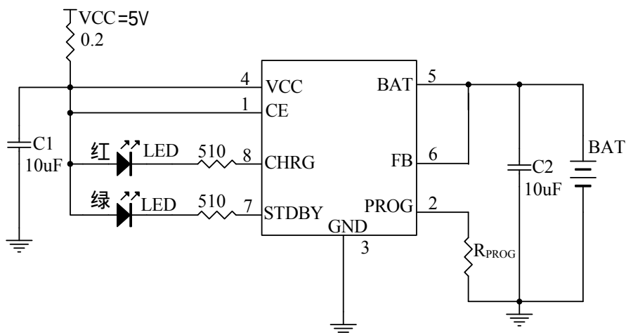
图 1 应用电路（恒定电压充电4.0V）
