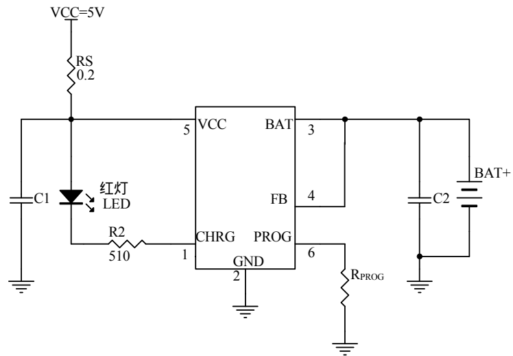
图1：应用电路（恒定电压充电4.0V）
