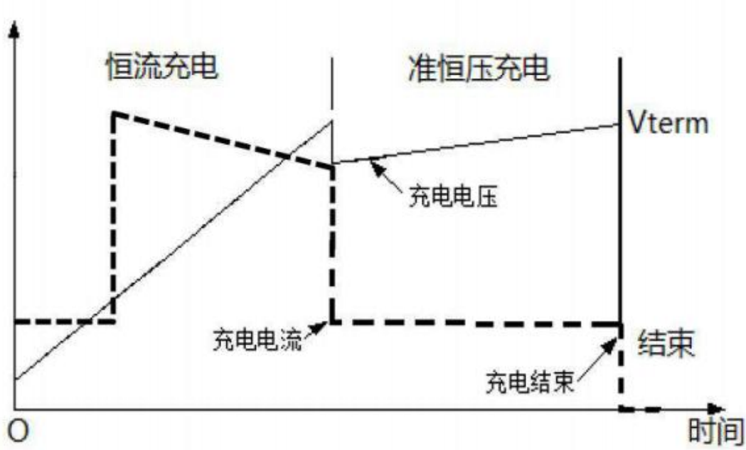
充电电流与电池电压关系图
