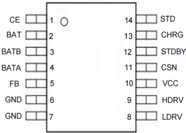
图 2 引脚图
