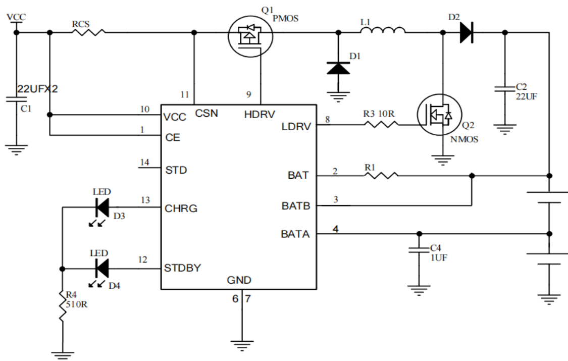
图 3 2节电池均衡充电应用图
