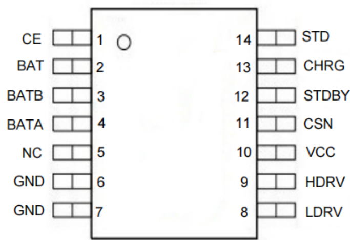
图 2 引脚图
